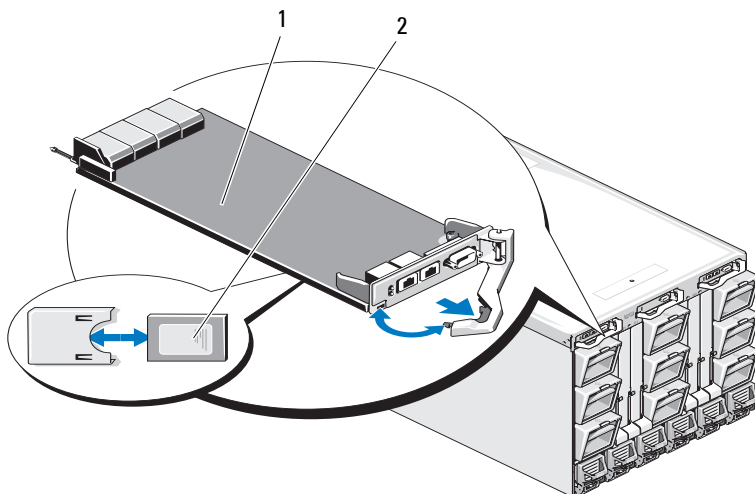
Figure 1-1. Installation et désinstallation de la carte SD module CMC
